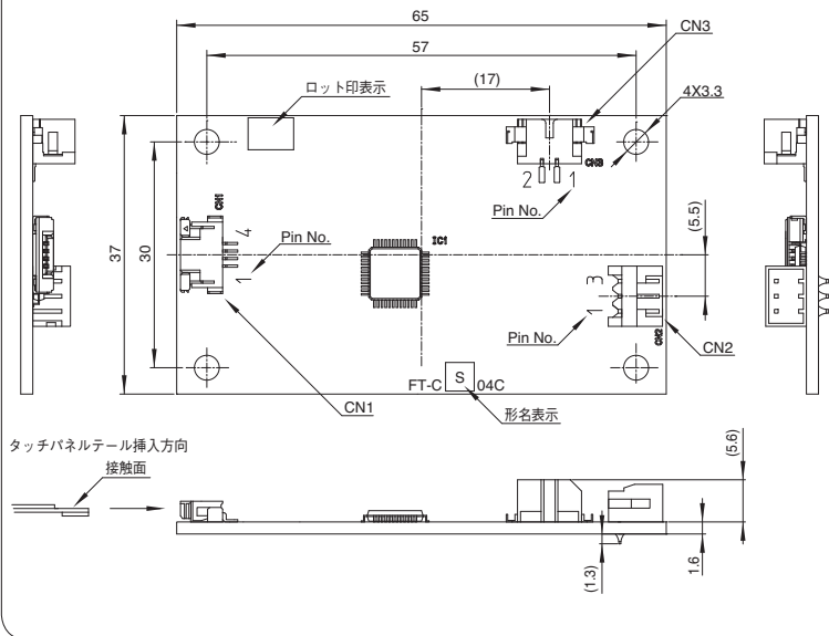
CN1 4線式アナログタッチパネル接続用 (4ピン)
