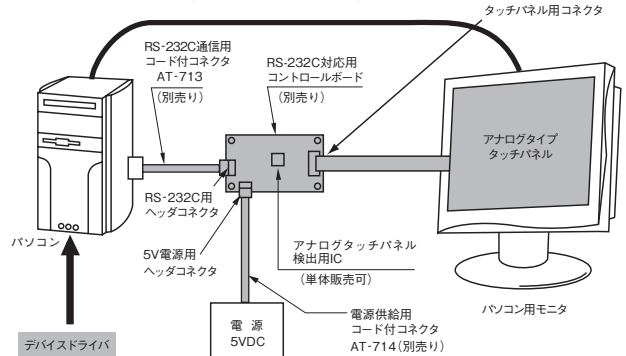
システム構成例(RS-232C対応用)
