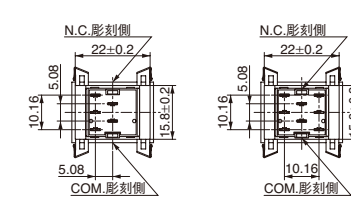
単極双投
