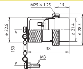
NCS-25 ■ -SP
