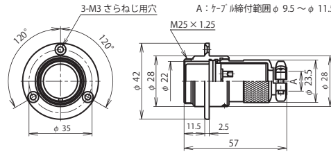
NCS-25 ■ -AdF(F)
