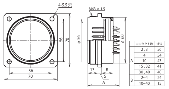
NCS-60 ■ -R
