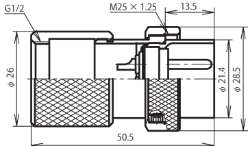
NCS-25 ■ -GPM 1/2 (注)
