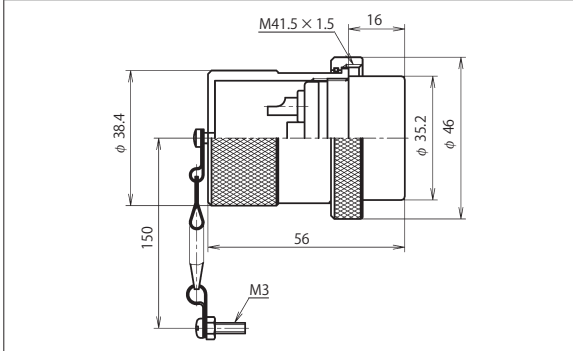
NCS-40 ■ -SP
