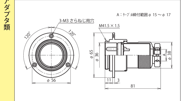
NCS-40 ■ -Ad(F)
