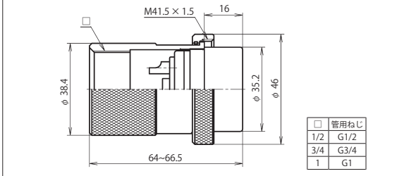
NCS-40 ■ -GP □ (注)
