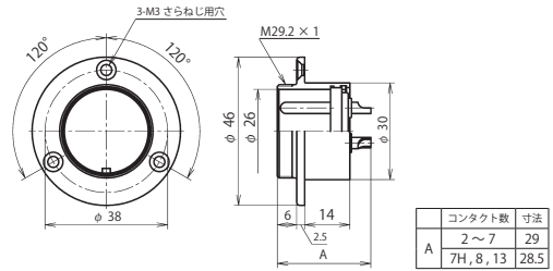
NCS-30 ■ -R
