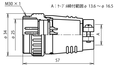
NJC-28 ■ -AdM
