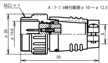
NJC-20 ■ -AdM
