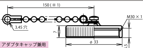
プラグキャップ: NJC-28-PCa
