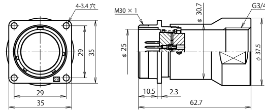
NJC-28 ■ -GAd(F)M3/4 (注)
