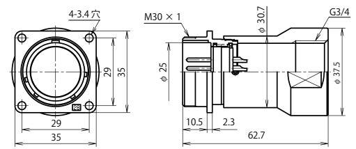
NJC-28 ■ -GAd(F)M3/4 (注)
