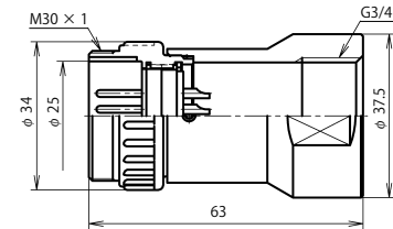
NJC-28 ■ -GAdM3/4 (注)
