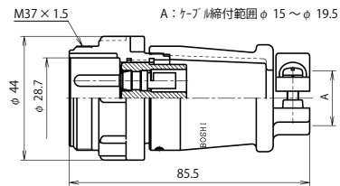
NJC-32 ■ -AdM
