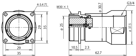
NJC-28 ■ -GAd(F)F3/4 (注)
