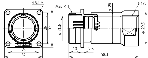
NJC-24 ■ -GAd(F)M1/2 (注)
