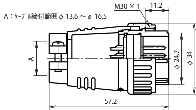
NJC-28 ■ -PM
