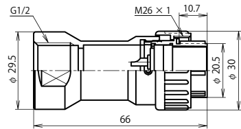
NJW-24 ■ -GPF1/2 (注)
