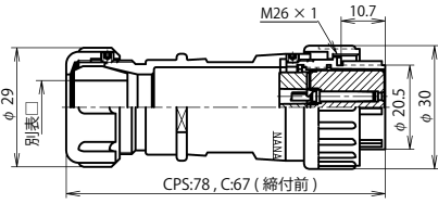
NJW-24 ■ -PF □
