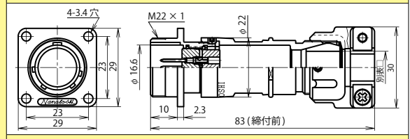
NJW-20 ■ -Ad(F)MK □
