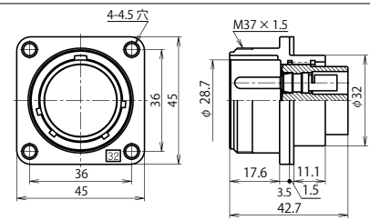
NJW-32 ■ -RM
