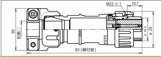
NJW-20 ■ -PFK □
