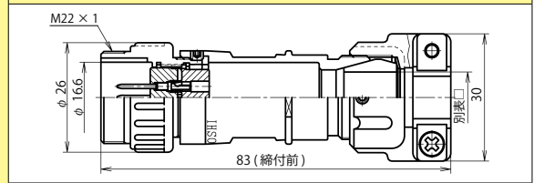
NJW-20 ■ -AdMK □
