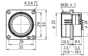
NJW-28 ■ -RM
