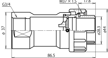
NJW-32 ■ -GPF3/4 (注)
