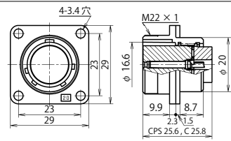
NJW-20 ■ -RF
