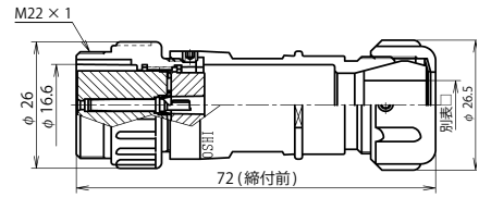
NJW-20 ■ -AdF □
