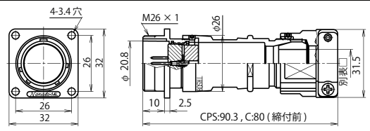
NJW-24 ■ -Ad(F)MK □
