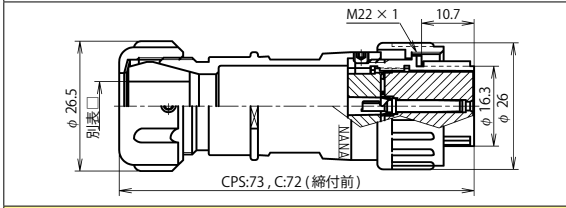
NJW-20 ■ -PF □
