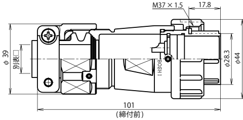
NJW-32 ■ -PF □
