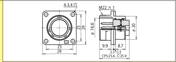
NJW-20 ■ -RM
