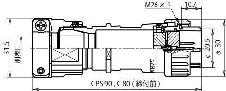
NJW-24 ■ -PMK □
