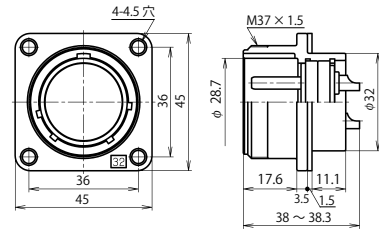
NJW-32 ■ -RM
