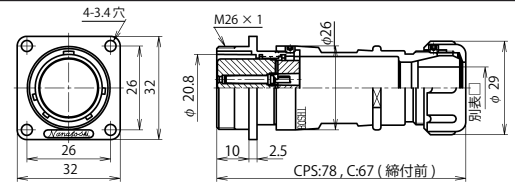
NJW-24 ■ -Ad(F)F □
