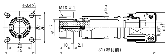
NJW-16 ■ -Ad(F)FK □
