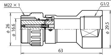
NJW-20 ■ -GAdF1/2 (注)
