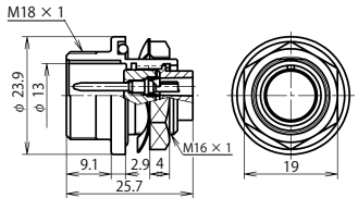
NJW-16 ■ -RBM
