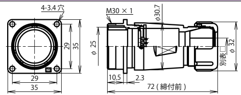
NJW-28 ■ -Ad(F)F □
