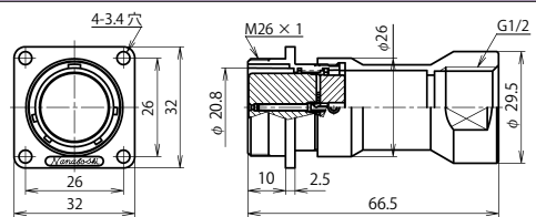
NJW-24 ■ -GAd(F)F1/2 (注)
