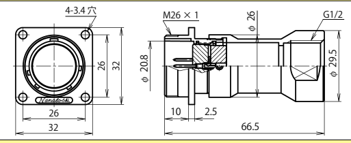
NJW-24 ■ -GAd(F)M1/2 (注)
