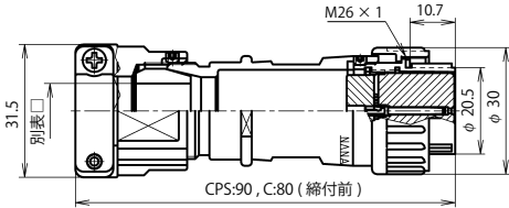
NJW-24 ■ -PFK □
