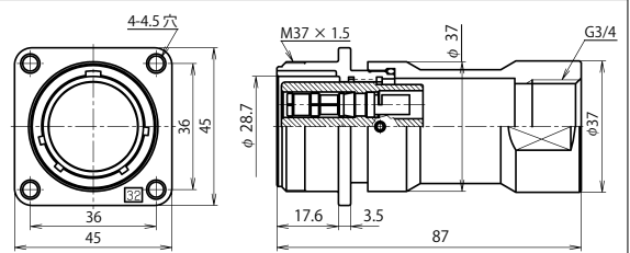
NJW-32 ■ -GAd(F)F3/4 (注)
