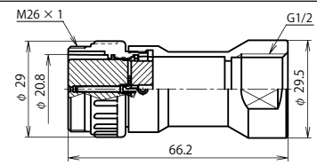
NJW-24 ■ -GAdF1/2 (注)
