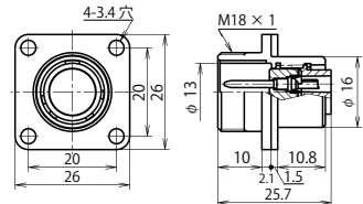
NJW-16 ■ -RM
