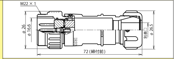
NJW-20 ■ -AdM □
