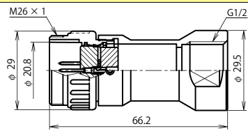
NJW-24 ■ -GAdM1/2 (注)
