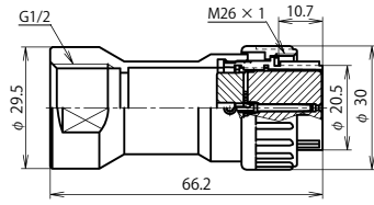
NJW-24 ■ -GPF1/2 (注)
