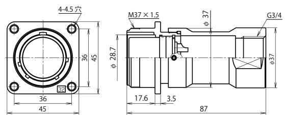
NJW-32 ■ -GAd(F)F3/4 (注)
