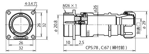
NJW-24 ■ -Ad(F)M □
