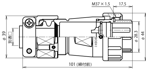
NJW-32 ■ -PM □
