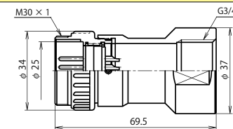
NJW-28 ■ -GAdM3/4 (注)
