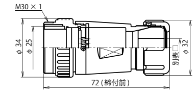
NJW-28 ■ -AdF □
