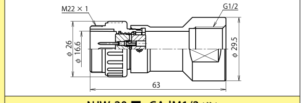
NJW-20 ■ -GAdM1/2 (注)
