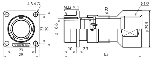
NJW-20 ■ -GAd(F)F1/2 (注)
