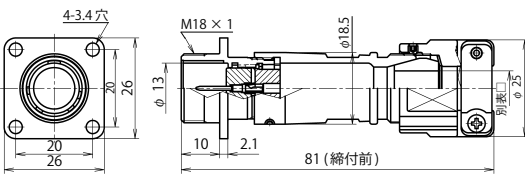
NJW-16 ■ -Ad(F)MK □
