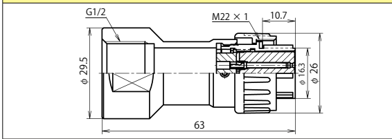
NJW-20 ■ -GPF1/2 (注)
