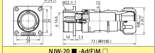
NJW-20 ■ -Ad(F)M □
