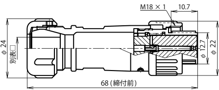
NJW-16 ■ -PF □
