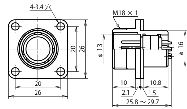
NJW-16 ■ -RM
