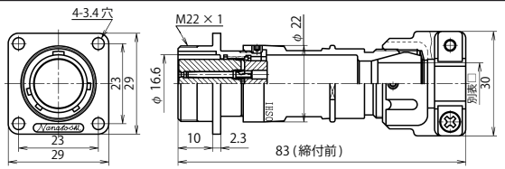
NJW-20 ■ -Ad(F)FK □
