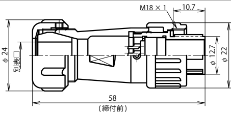
NJW-16 ■ -PF □
