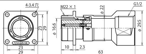
NJW-20 ■ -GAd(F)F1/2 (注)
