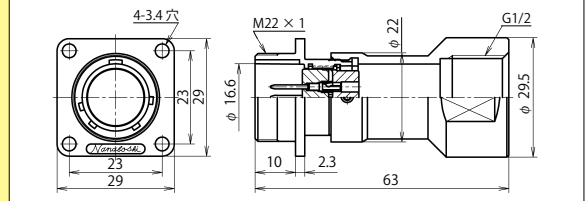
NJW-20 ■ -GAd(F)M1/2 (注)
