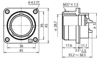
NJW-32 ■ -RF
