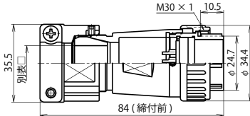
NJW-28 ■ -PFK □
