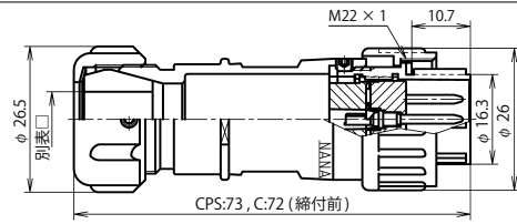
NJW-20 ■ -PM □
