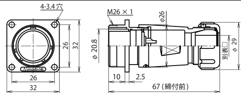
NJW-24 ■ -Ad(F)F □
