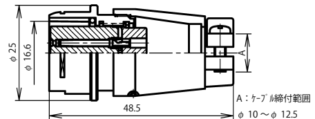
NR-20 ■ -AdF
