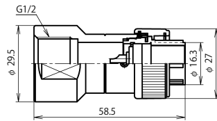
NR-20 ■ -GPF1/2 (注)
