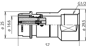
NR-20 ■ -GAdF1/2 (注)
