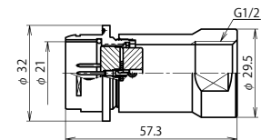
NR-24 ■ -GAdM1/2 (注)
