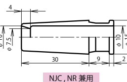
ケーブルブッシング: NJC-20-CB
