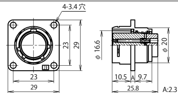
NR-20 ■ -RF
