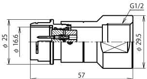
NR-20 ■ -GAdM1/2 (注)
