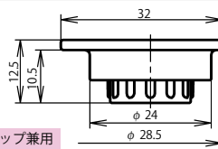
レセプタクルキャップ: NR-20-RCa・1
