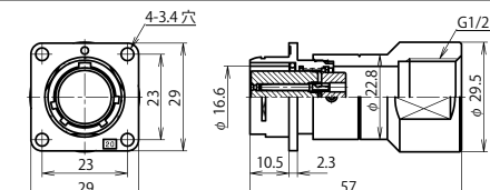
NR-20 ■ -GAd(F)F1/2 (注)
